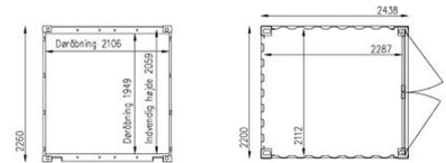
8 fods standard stålcontainer
